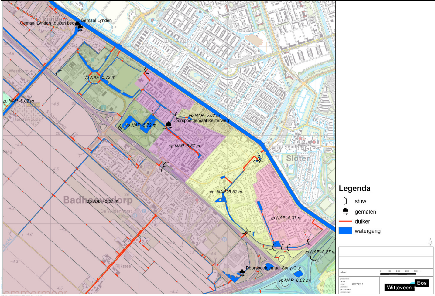
Afbeelding I.7.1. Overzicht watersysteem Badhoevedorp (vp: vastpeil; zp: zomerpeil)
