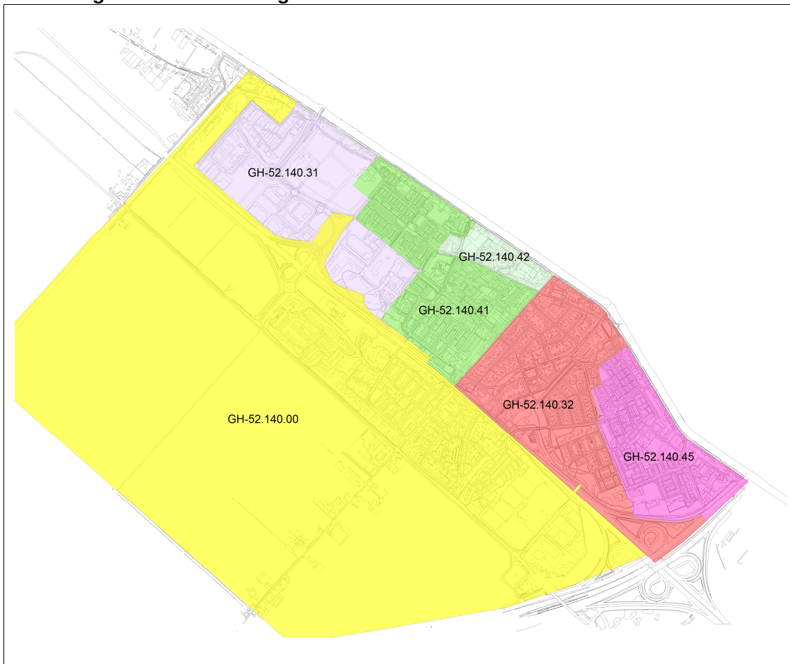
Afbeelding 5.8. Peilvakindeling
