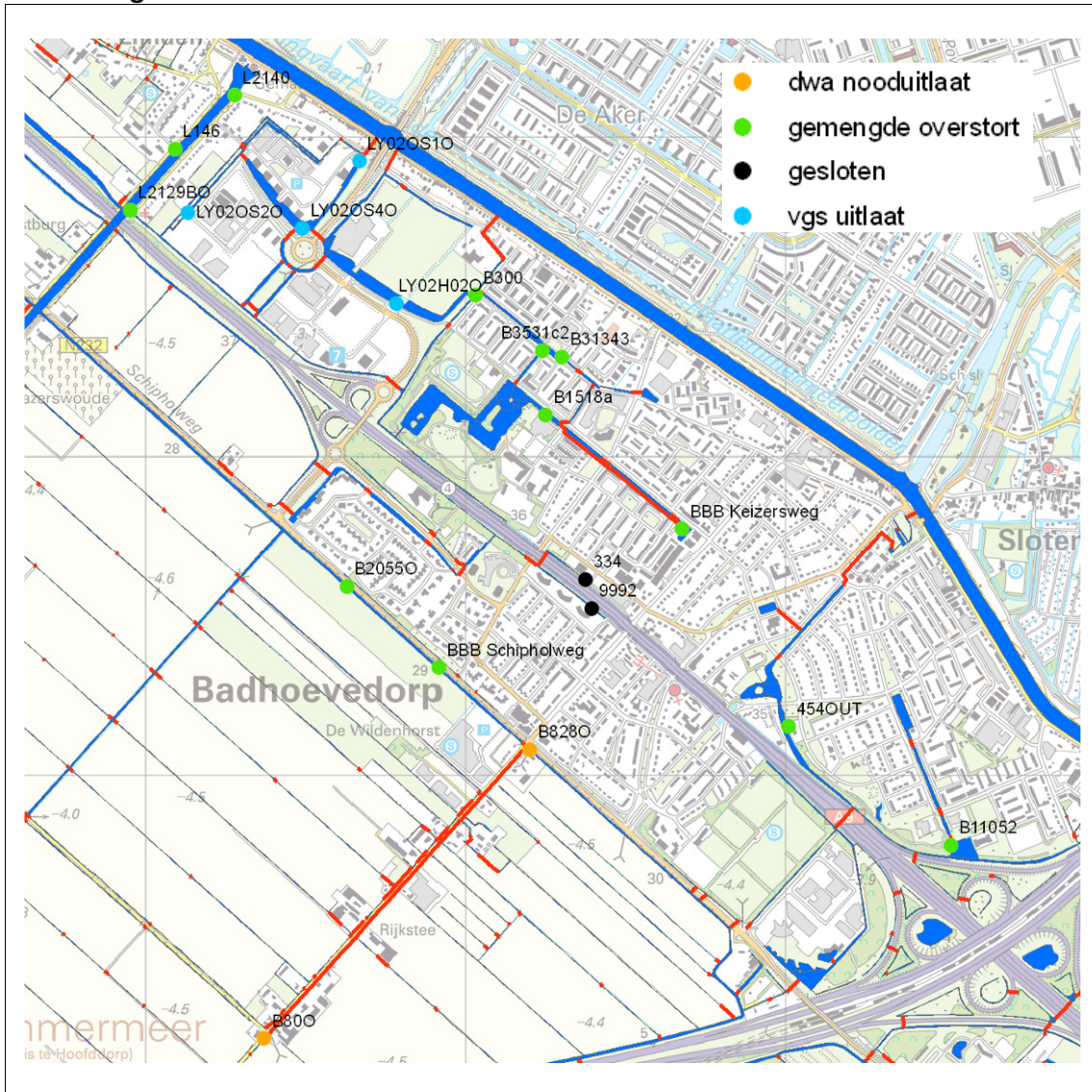
Afbeelding 2.10. Overstortlocaties
