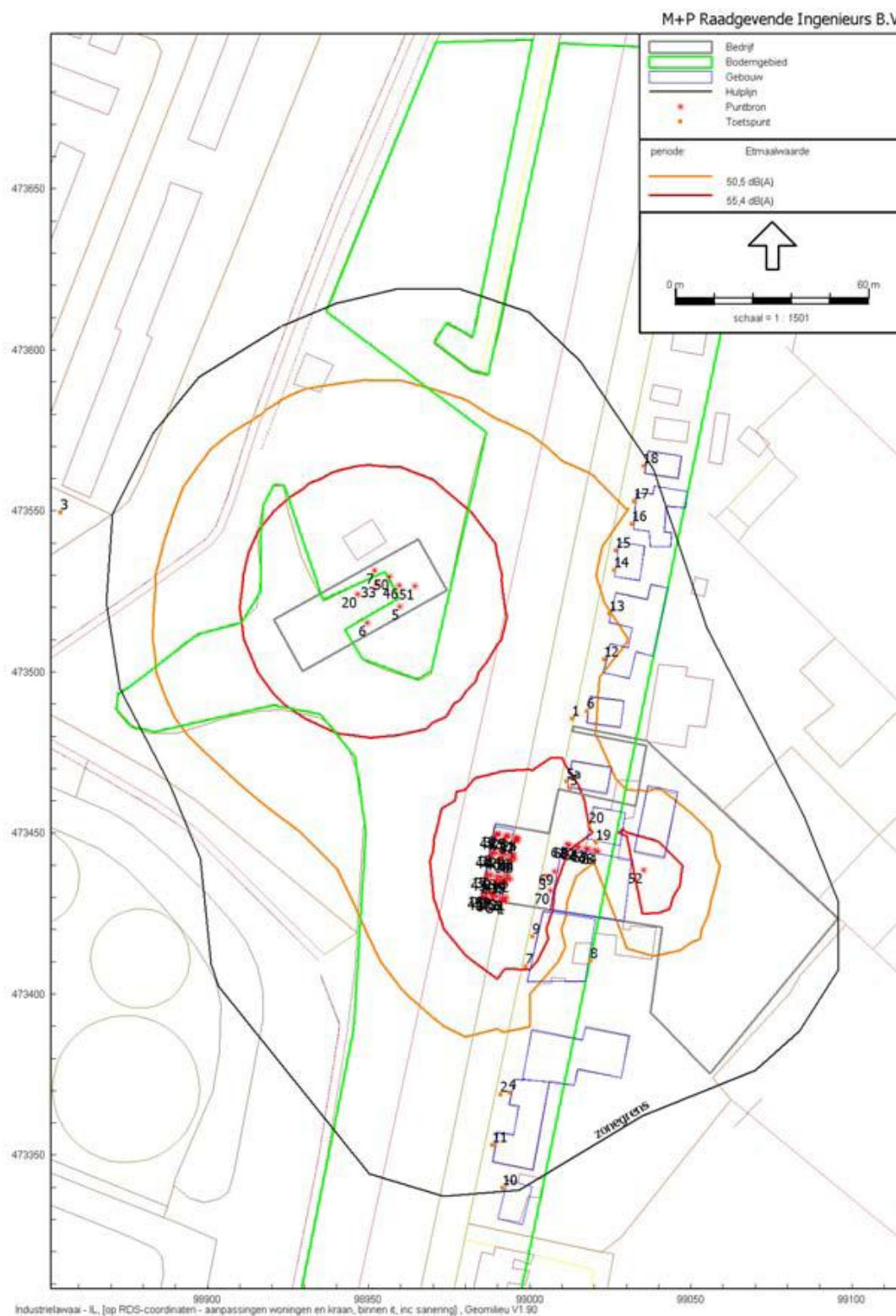
Figuur: zonegrens (zwart) en berekende 50 dB(A)-contour (oranje) bij aangewezen industrieterrein
